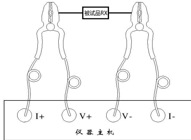
图二 接线图
